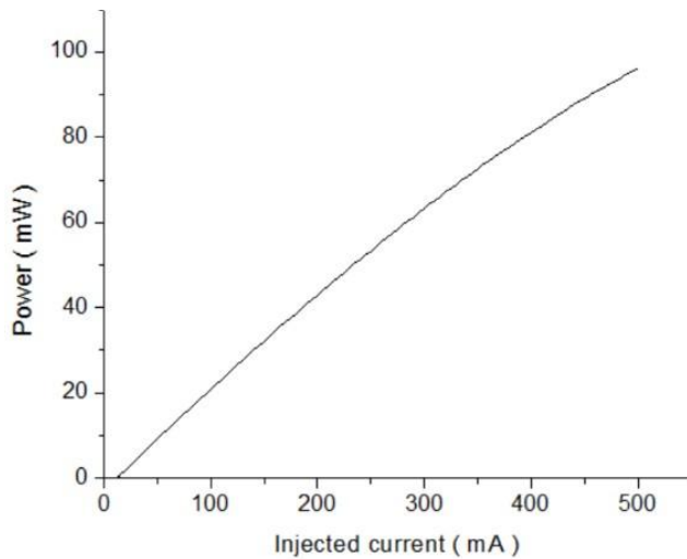
Laser P-I
